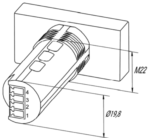
Рисунок А.2 – Габаритный чертеж корпуса прибора. Вид сзади
