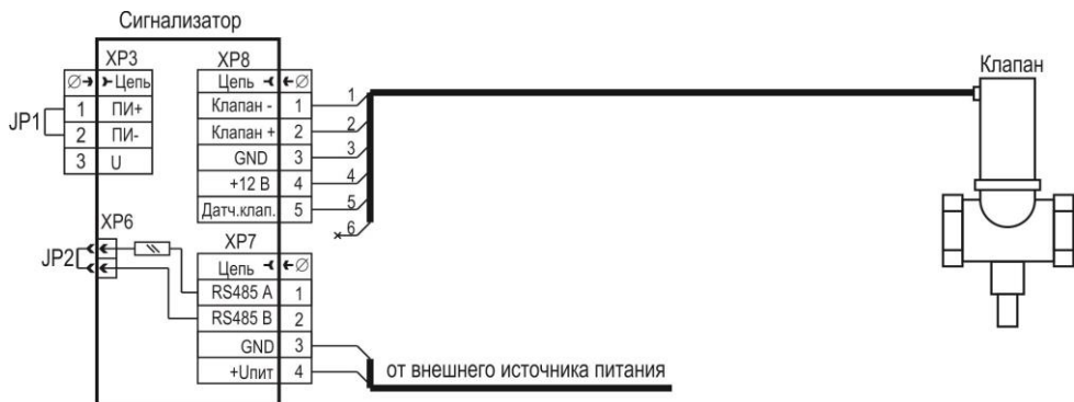
Рисунок В.3 – Схема подключения сигнализатора СЗ-2ЕВ
