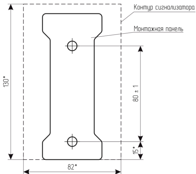
Рисунок Б.1 – Монтажные размеры
