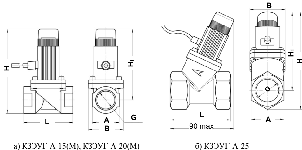
Рисунок 1 – Внешний вид клапанов
